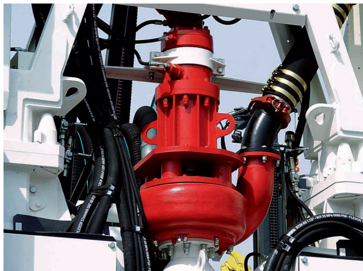
Специальное исполнение "Habermann" - "KBKT-V1" с гидравлическим приводом, оснащающий траншеекопатели ведущих европейских специализированных производителей
