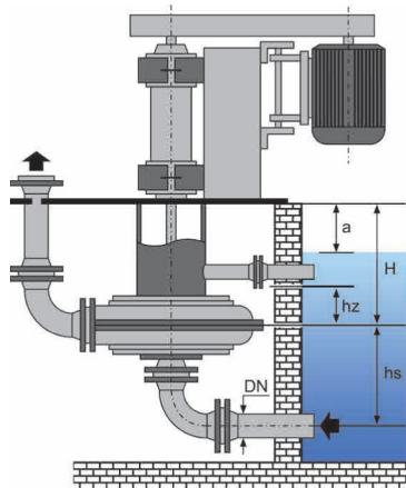
Сухая установка V310
